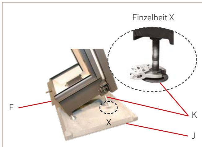
Abb. 31: Kamineinsatz nach vorn kippen und Stellfüße einstellen
