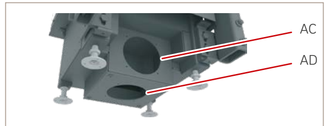
Abb. 35: Anschlussöffnungen Verbrennungszuluft
