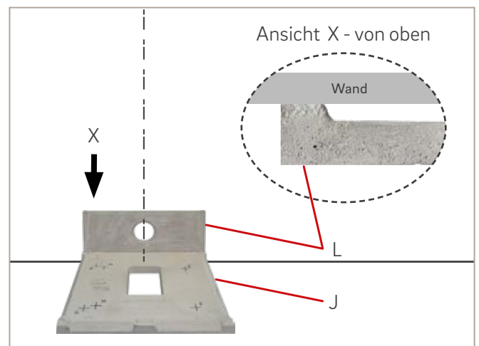
Abb. 17: Rückwand 1 setzen
