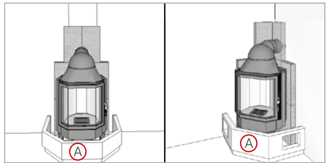
Abb. 9: S4 Front/S4 Eck Montage Unterbauteil
