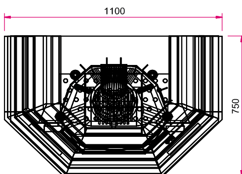
Draufsicht mit Abgang oben M 1:20
