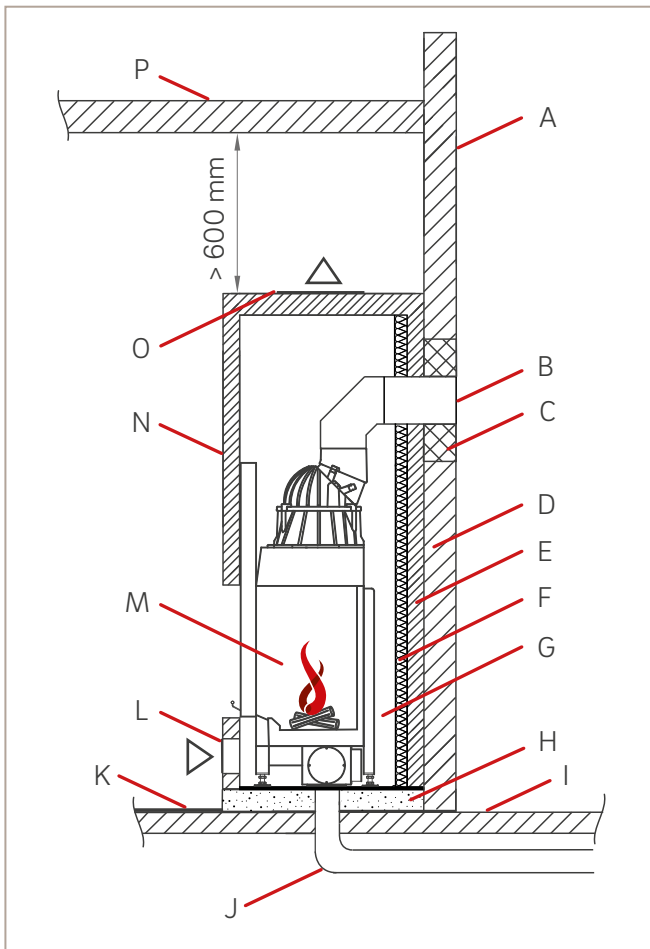
Abb. 25: Einbaubeispiel für eine Systemanlage vor zu schützenden Wänden, Böden, Decken
