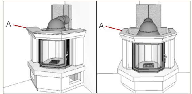
Abb. 13: S4 Front/S4 Eck Montage Sturz
