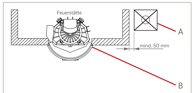
Abb. 28: Schutz und Abstände bei beheizten Flächen
