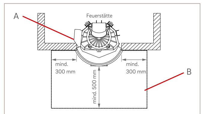
Abb. 26: Fußbodenschutz im Bereich vor der Feuerraumöffnung
