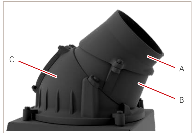
Abb. 6: Gusskuppel, Position 45°
