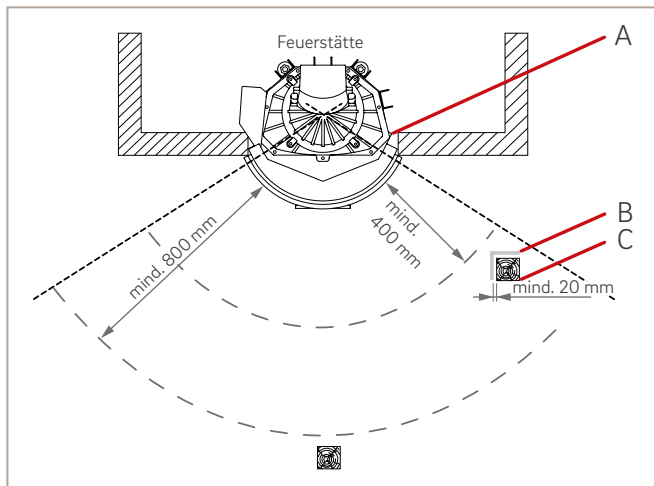
Abb. 27: Schutz von brennbaren Bauteilen im Strahlungsbereich vor der Feuerraumöffnung
