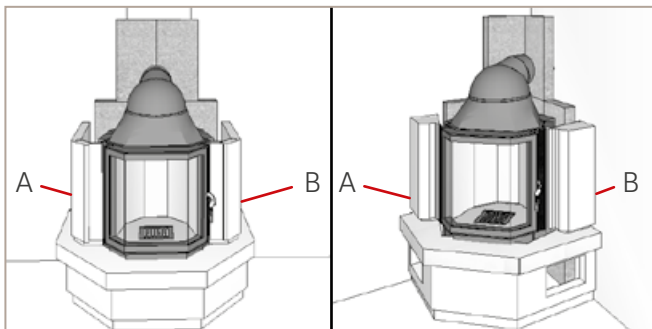
Abb. 12: S4 Front/S4 Eck Montage Seitenteile links/rechts
