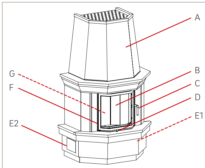
Abb. 2: Abbildung S4 Front
