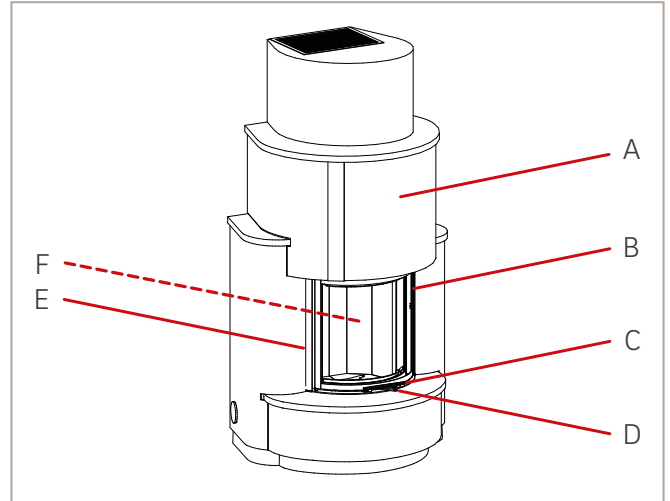
Abb. 3: Abbildung S5 Front hochschiebbar
