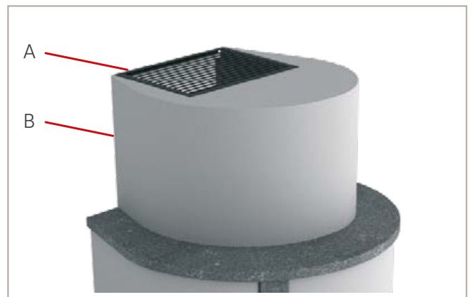
Abb. 35: Deckengitter einsetzen
