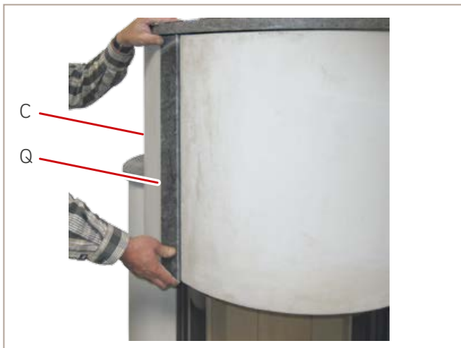
Abb. 33: Naturstein-Frontblende ankleben
