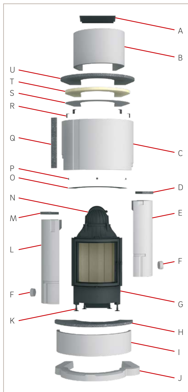
Abb.7: Aufbau S5 Front
