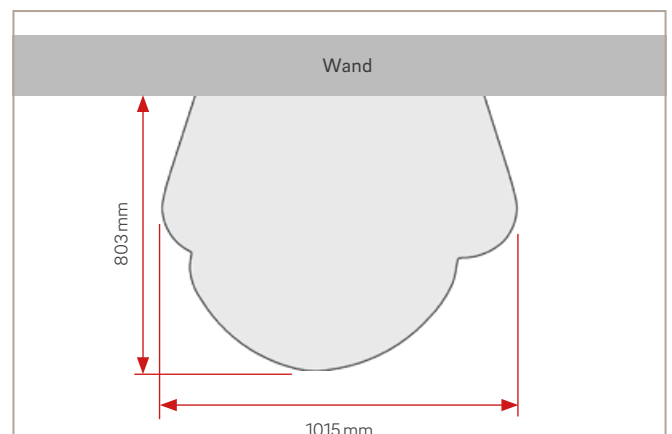
Abb. 9: Estrichaussparung
