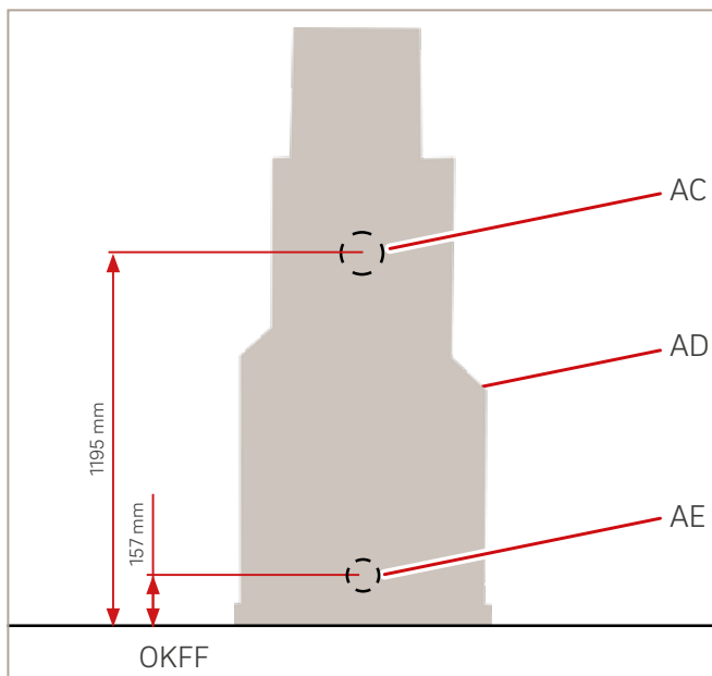
Abb. 29: Anschlüsse an der Dämmung anzeichnen und bohren, schematische Darstellung
