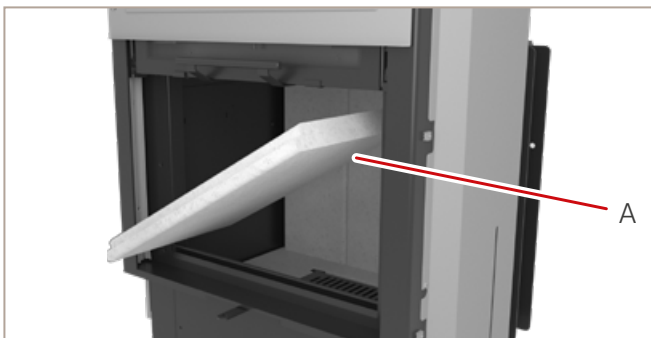
Abb. 44: seitliche Innenauskleidung entnehmen
