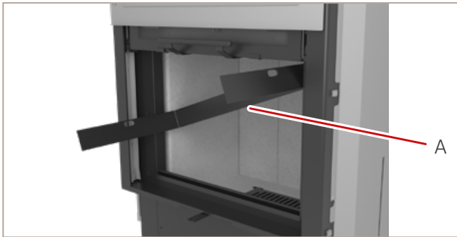
Abb. 43: Halter entnehmen
