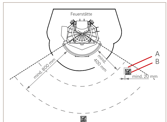
Abb. 54: Schutz von brennbaren Bauteilen im Strahlungsbereich vor der Feuerraumöffnung
