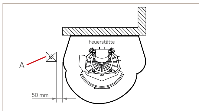
Abb.55: Schutz und Abstände bei beheizten Flächen
