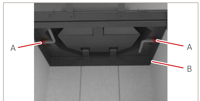
Abb. 42: Befestigungsschrauben lösen
