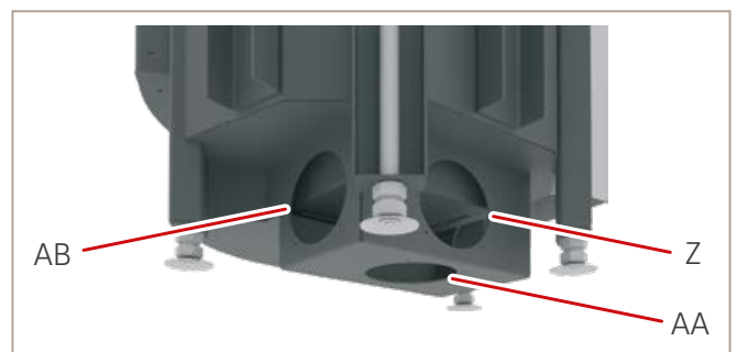
Abb. 15: Anschlussöffnung Verbrennungszuluft
