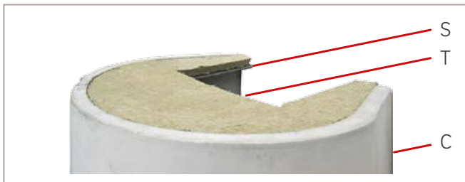
Abb. 25: Dämmwolle platzieren
