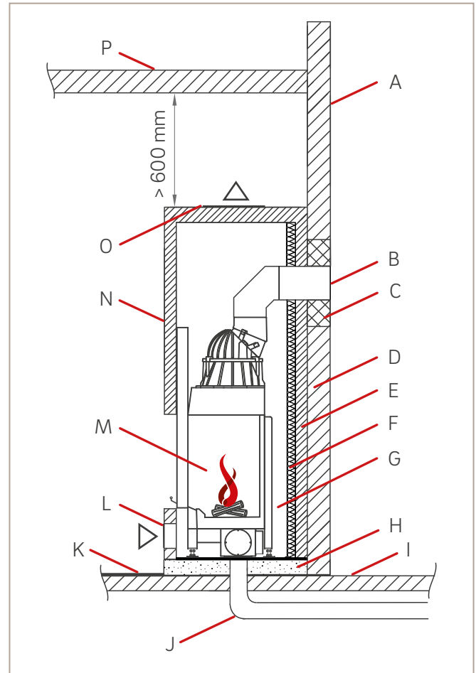
Abb. 52: Einbaubeispiel für eine Systemanlage vor zu schützenden Wänden, Böden, Decken
