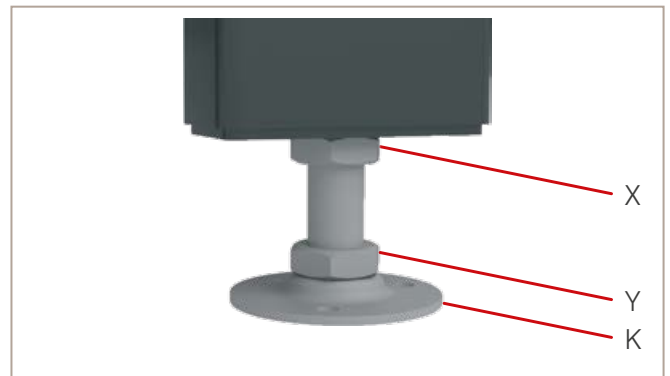
Abb.12: Stellfuß mit Muttern
