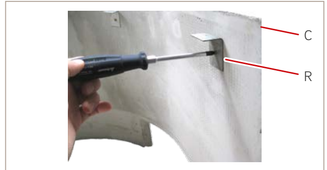
Abb. 21: Auflegewinkel Trägerplatte Dämmung anbringen
