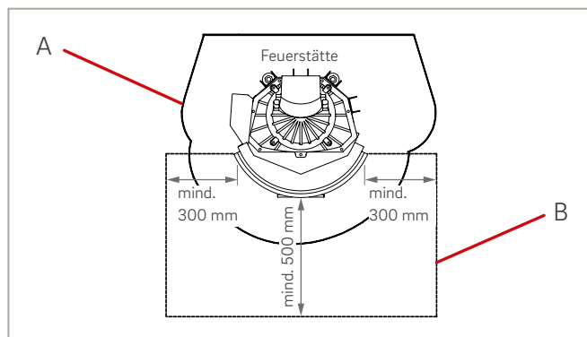
Abb. 53: Belag aus nicht brennbaren Baustoffen im Bereich vor der Feuerraumöffnung
