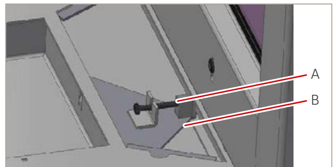
Abb. 56: Befestigungsschraube lösen
