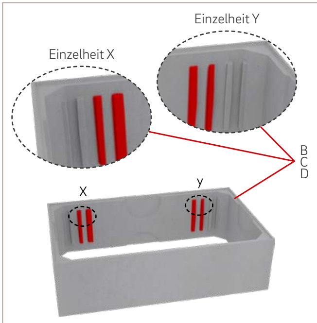
Abb. 44: Oberbauteil Rippen entfernen
