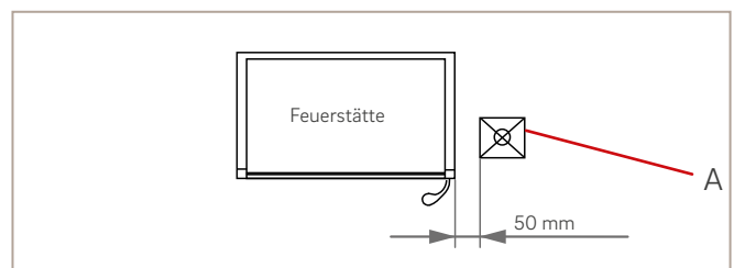
Abb. 75: Schutz und Abstände bei beheizten Flächen
