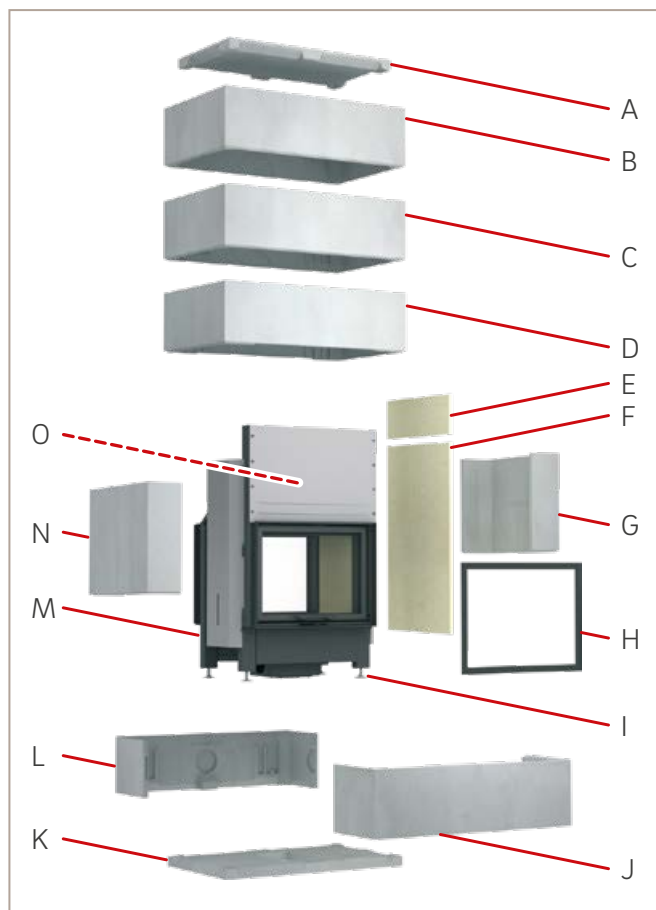
Abb. 29: Aufbau am Beispiel S7 TV Hoch
