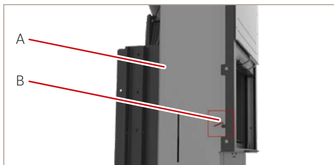
Abb. 57: Demontage Gewichtsschachtabdeckungen
