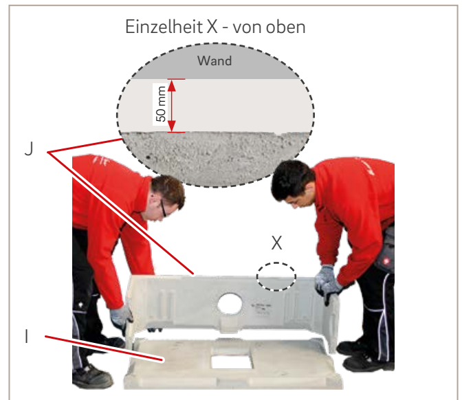
Abb. 10: Unterbauteil hinten setzen
