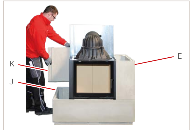
Abb.21: Rückwand setzen
