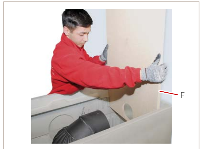
Abb.50: Dämmplatten einsetzen und Anschluss markieren
