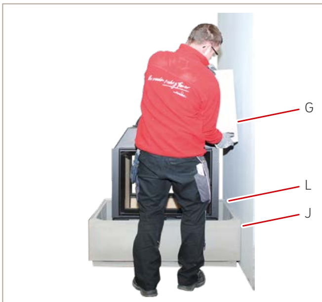
Abb. 42: Seitenteil rechts setzen
