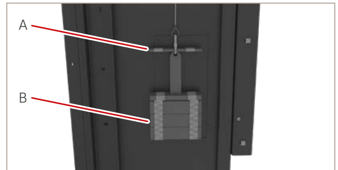
Abb. 59: Ausgleichsgewichte entnehmen
