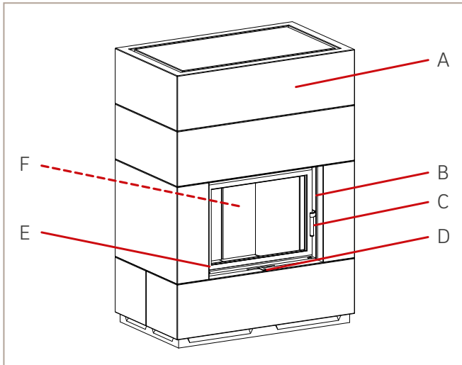
Abb. 2: Abbildung S7 Kurz schwenkbar
