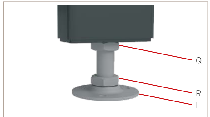
Abb. 35: Stellfuß mit Muttern
