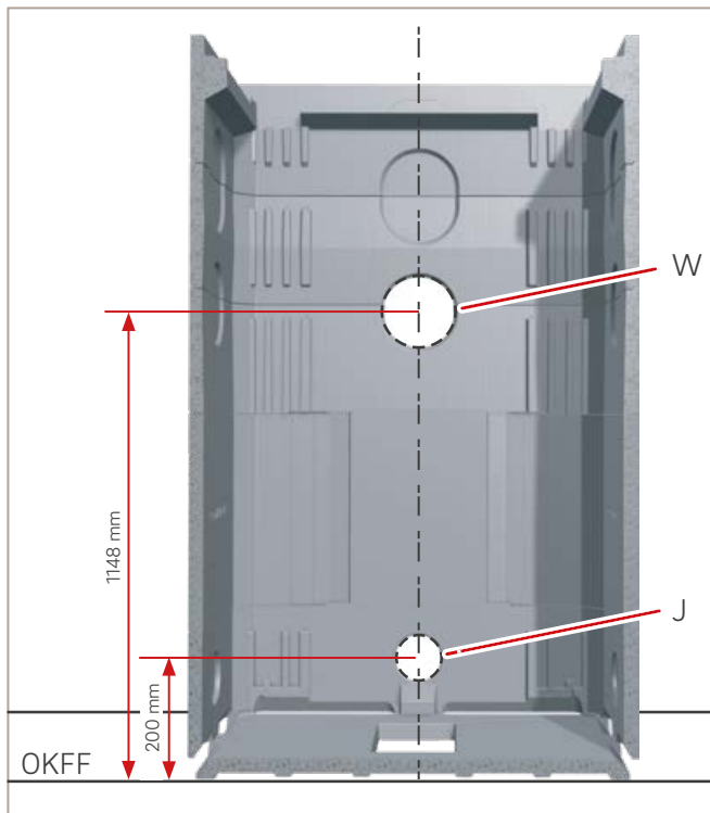
Abb. 26: Anschlüsse an der Zimmerwand anzeichnen und bohren, schematische Darstellung
