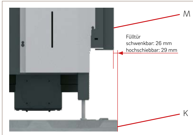
Abb. 37: Kamineinsatz ausrichten
