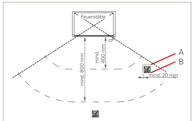
Abb. 74: Schutz von brennbaren Bauteilen im Strahlungsbereich vor der Feuerraumöffnung
