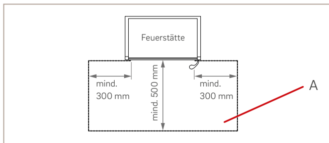
Abb. 73: Belag aus nicht brennbaren Baustoffen im Bereich vor der Feuerraumöffnung
