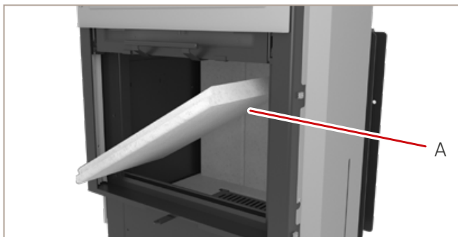
Abb. 62: seitliche Innenauskleidung entnehmen
