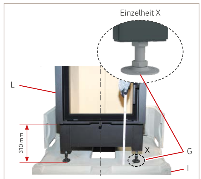
Abb. 14: Kamineinsatz auf Bodenplatte setzen
