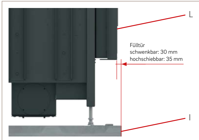
Abb. 15: Kamineinsatz ausrichten
