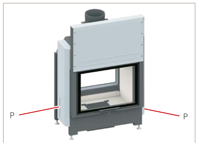
Abb.33: Position Feststellschrauben am Kamineinsatz
