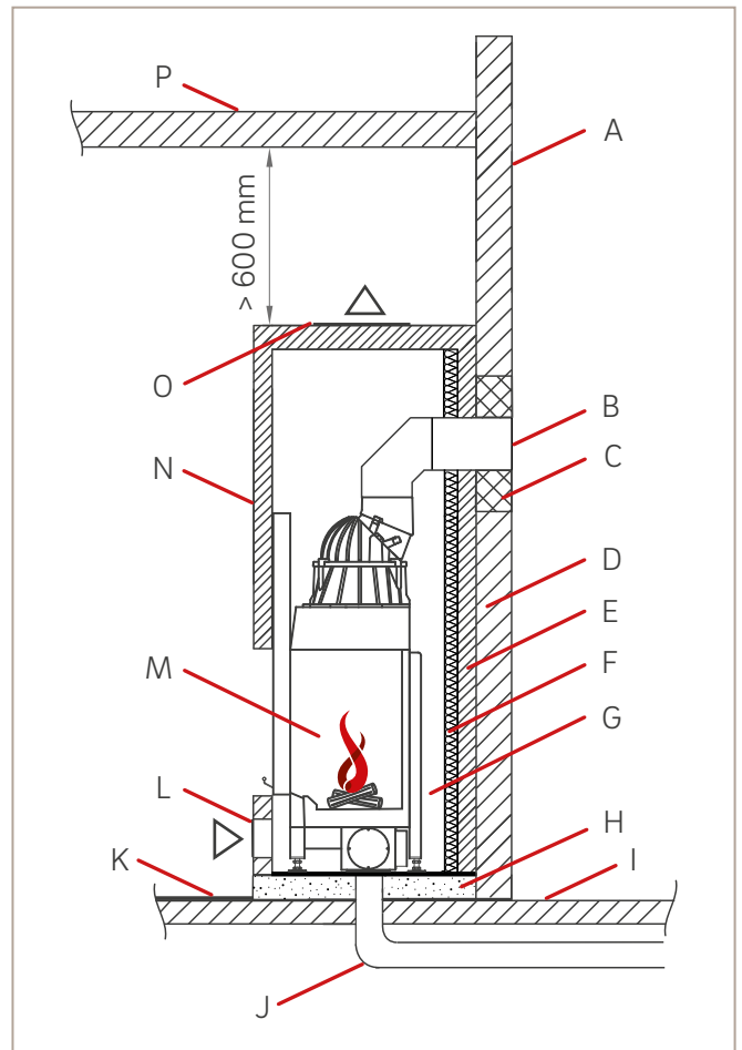
Abb. 72: Einbaubeispiel für eine Systemanlage vor zu schützenden Wänden, Böden, Decken
