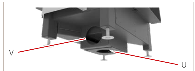
Abb. 40: Anschlussöffnung Verbrennungszuluft
