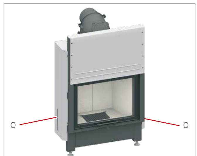
Abb. 11: Position Feststellschrauben am Kamineinsatz
