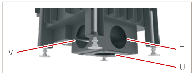
Abb. 18: Anschlussöffnung Verbrennungsluft
