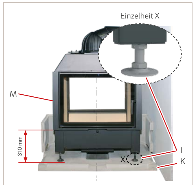
Abb. 36: Kamineinsatz auf Bodenplatte setzen
