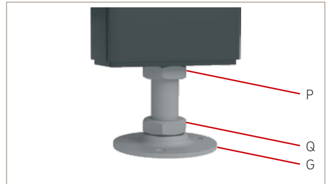
Abb. 13: Stellfuß mit Muttern
