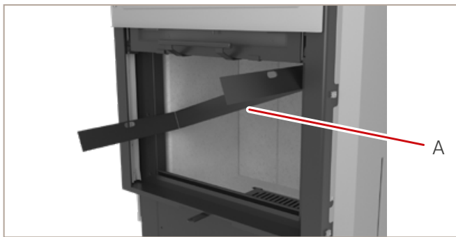
Abb. 61: Halter entnehmen
