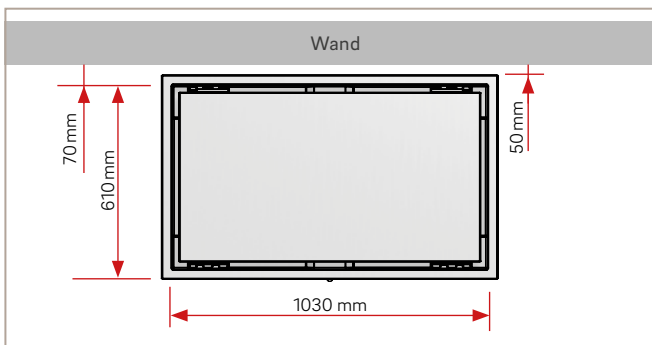
Abb. 9: Estrichaussparung
