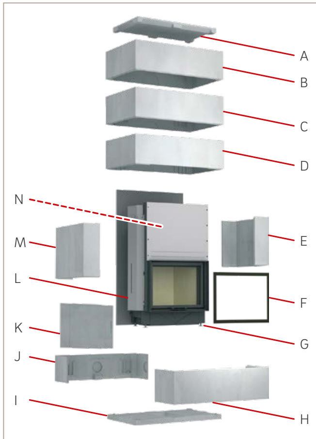
Abb. 7: Aufbau am Beispiel S7 Hoch
