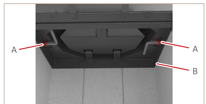
Abb. 60: Befestigungsschrauben lösen
