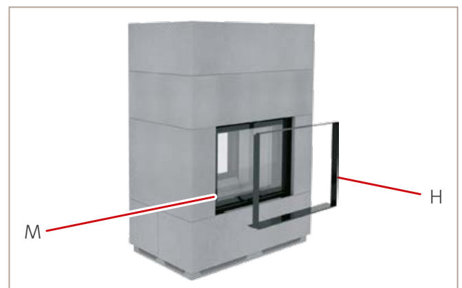
Abb. 53: Blendrahmen positionieren
