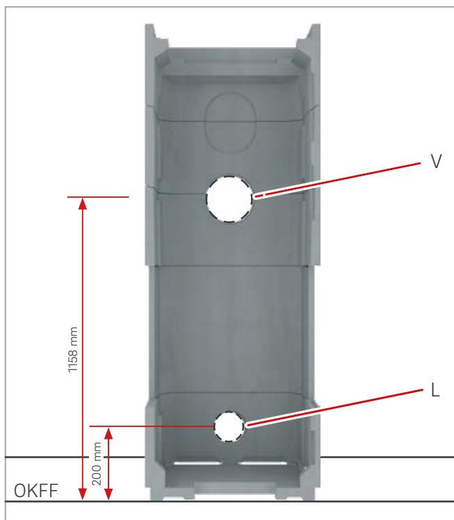
Abb. 51: Anschlüsse an der Zimmerwand anzeichnen und bohren, schematische Darstellung
