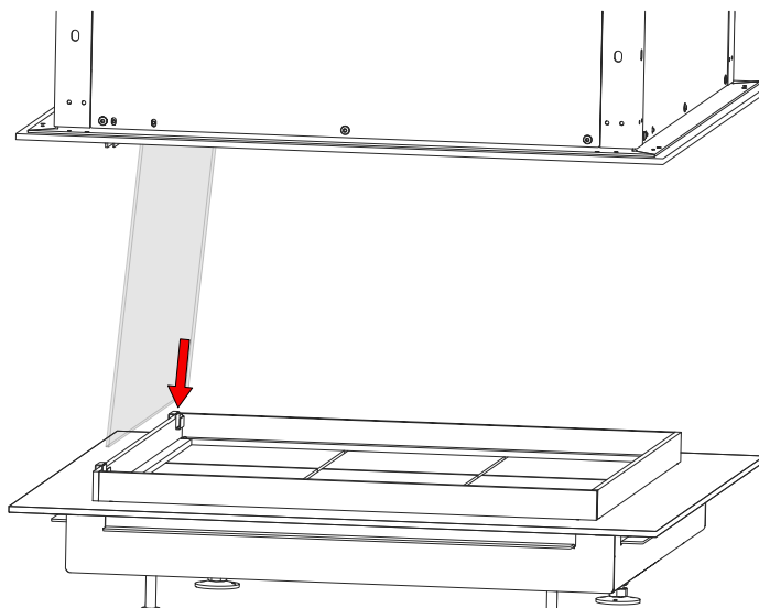
Abb. 2: Glas einsetzen
