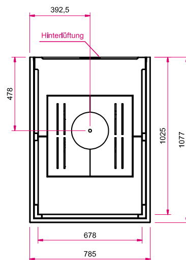
Draufsicht M 1:25
