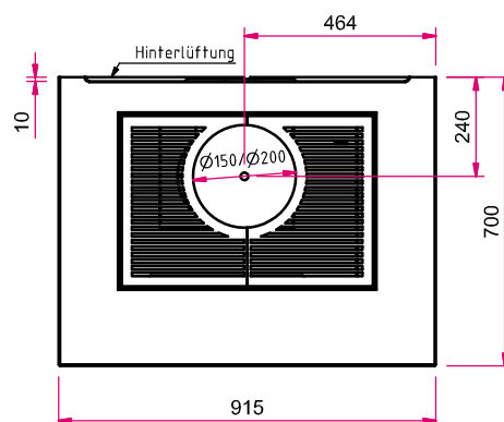
Draufsicht M 1:20
