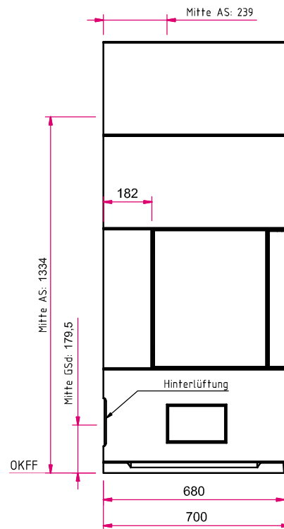
Seitenansicht links M 1:20
