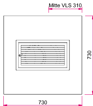
Draufsicht M 1:20
