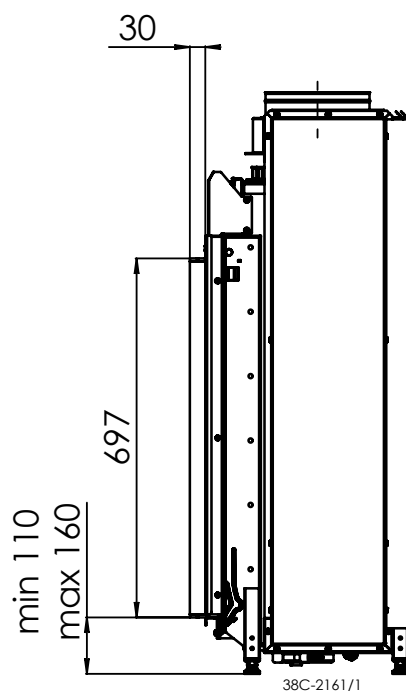
Maestro 75 RCH
