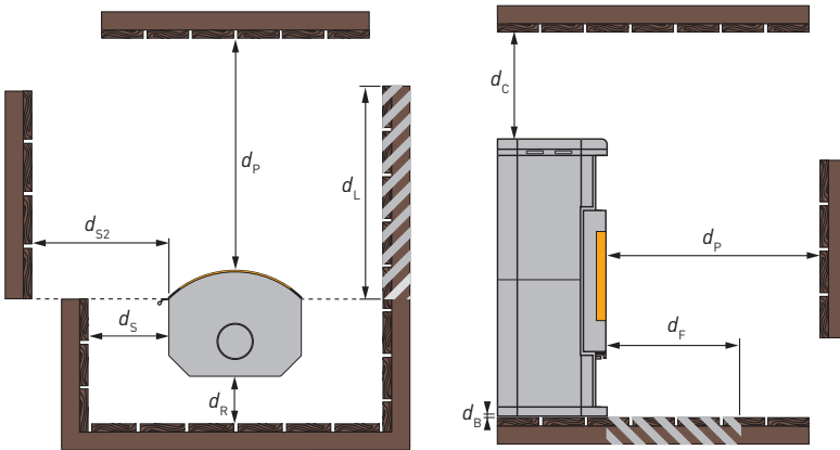
Draufsicht Brennkammer
