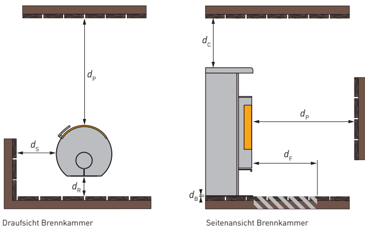
Draufsicht Brennkammer
