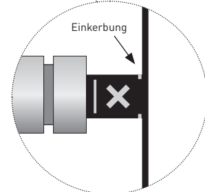
Abb. 4.5 Verbrennungsluftregler Betriebsphase
